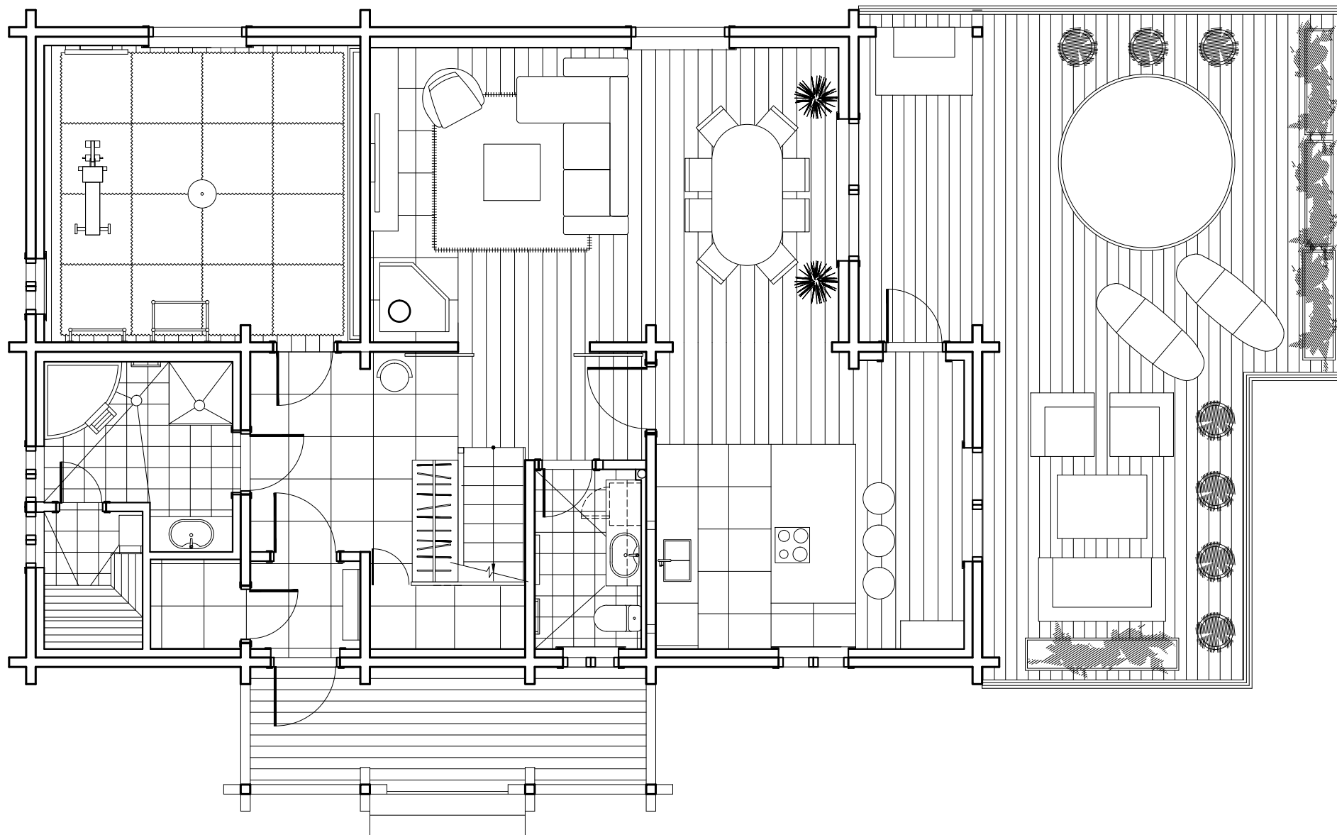
План 1 этажа.
