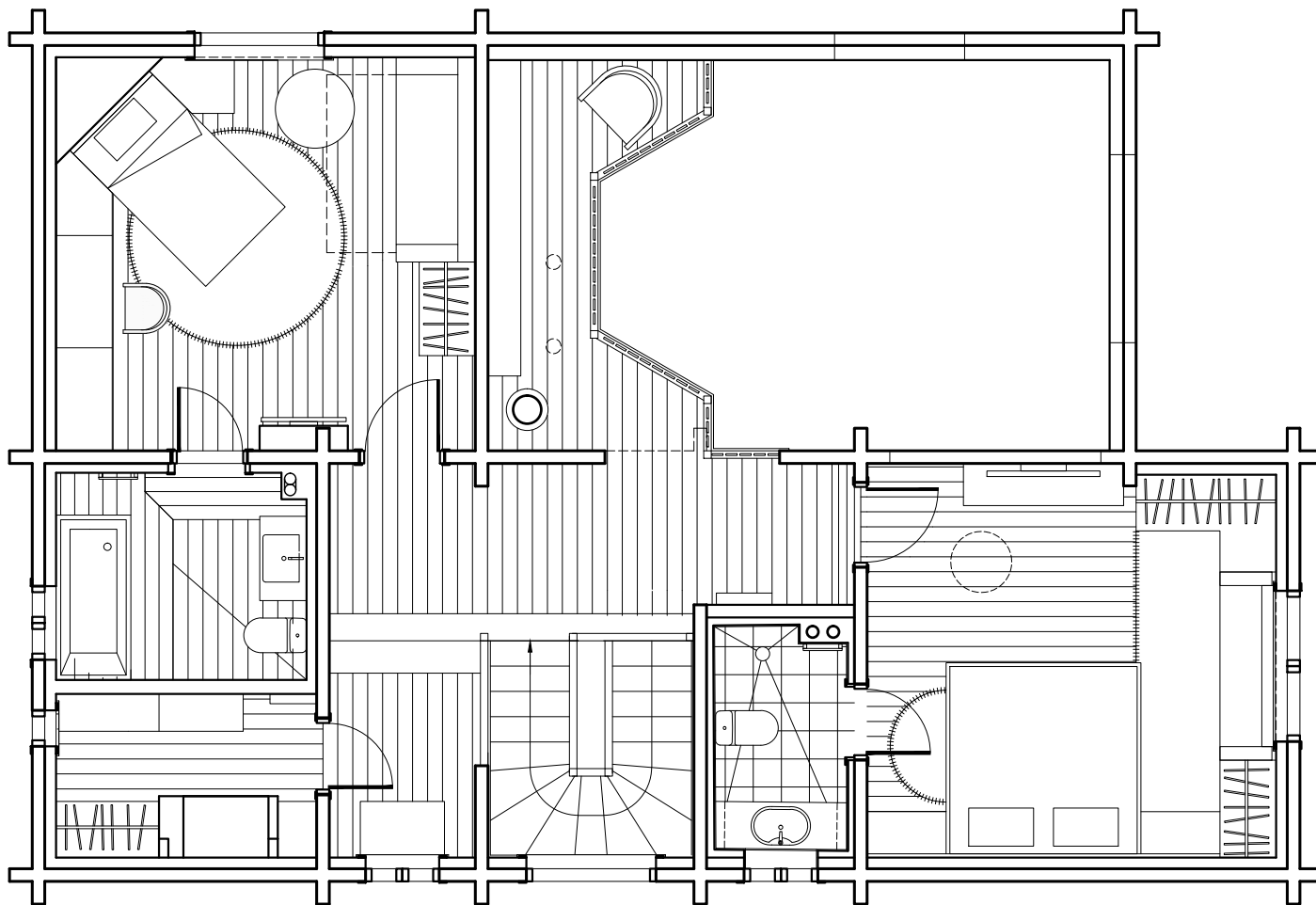
План 2 этажа.
